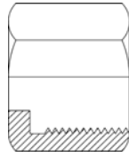
Flare Tube Nut
