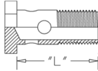
F15 - R/M BSPP / Metric Banjo Bolt Page 21
