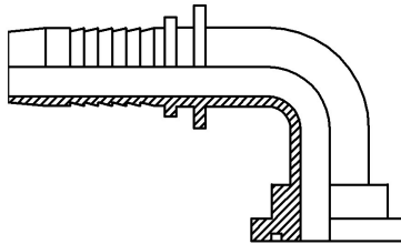
Code 61 Flange 90°
