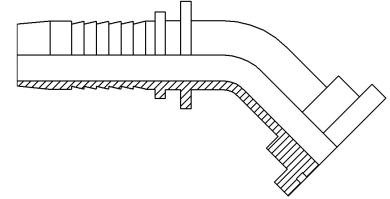
Code 61 Flange 45°
