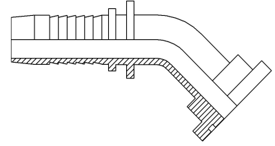
Code 62 Flange 45°
