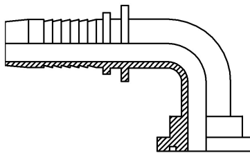
Code 62 Flange 90°
