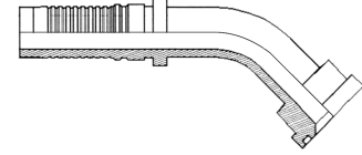
Code 61 Flange 45° Interlock
