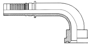
Code 61 Flange 90° Interlock
