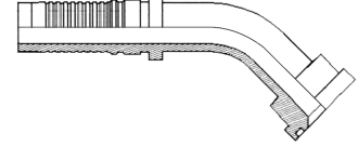
Code 62 Flange 45° Interlock
